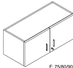
Colgante 2P F: 75/80/90 P: 40 H: 40
