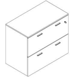
Bajo 2K F: 75/80/90 P: 50 H: 75
