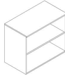
Bajo Abierto F: 75/80/90 P: 50 H: 75
