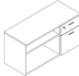
Lateral Fija/Móvil 1C1K1R Izquierda o Derecha F: 120 P: 45 H: 51,5/55 Frente cajón: 42
